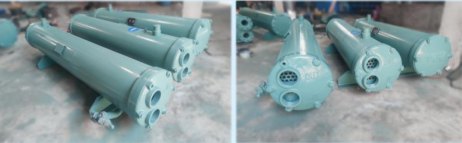
15. Sản xuất bình ngưng, KH công ty CP Kỹ nghệ xanh Việt Nam, CN tại huyện Điện Bàn, tỉnh Quảng Nam
