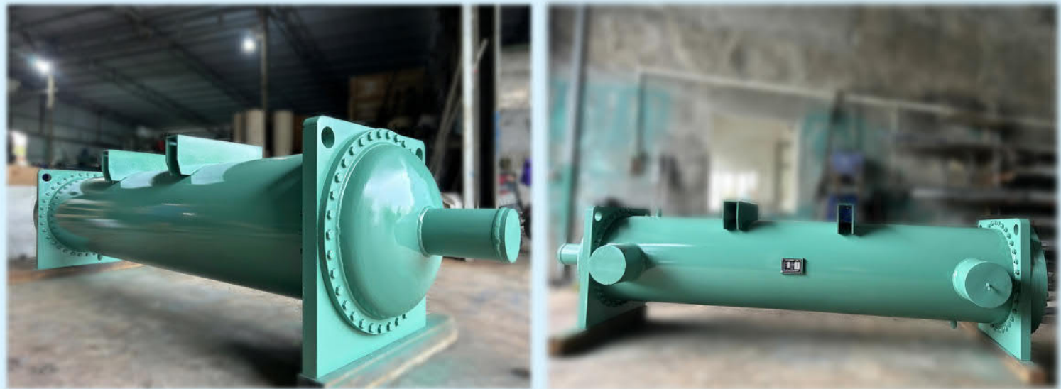
13. Sản xuất bình bay hơi 75Hp, vỏ inox, KH công ty Cơ điện lạnh Phong Thịnh, phường Phú Thạnh, Tân Phú, Tp. HCM - Dùng cho ngành thực phẩm.
